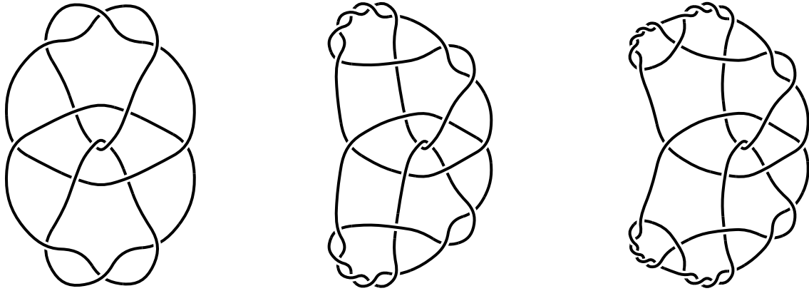
Fig. 6: The links LL_2(1) , LL_2(2) , LL_2(3)
